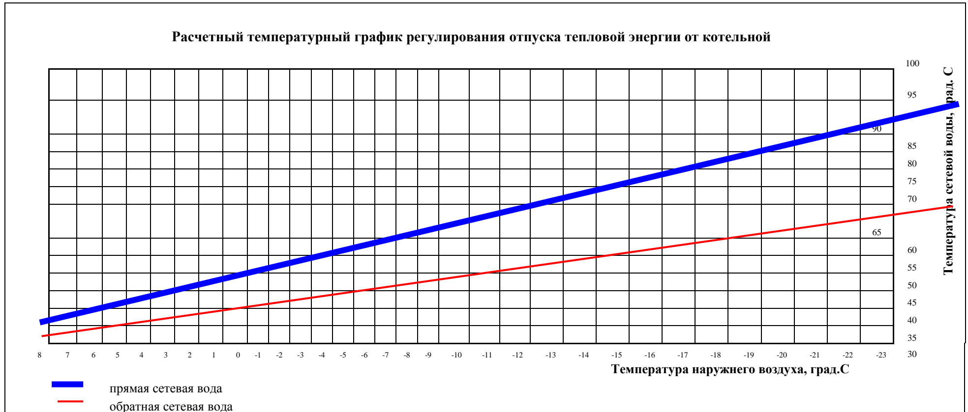
Рис.5.2. Расчетный температурный график регулирования отпуска тепловой энергии от котельной
